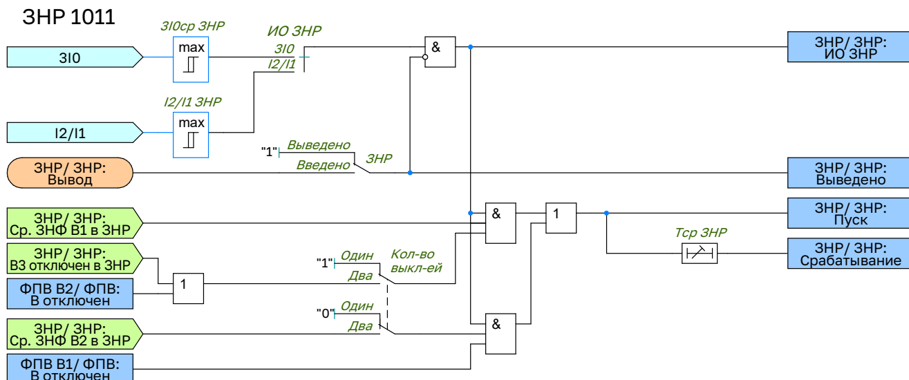
Рисунок 2.12 – Функциональная схема логики ЗНР
